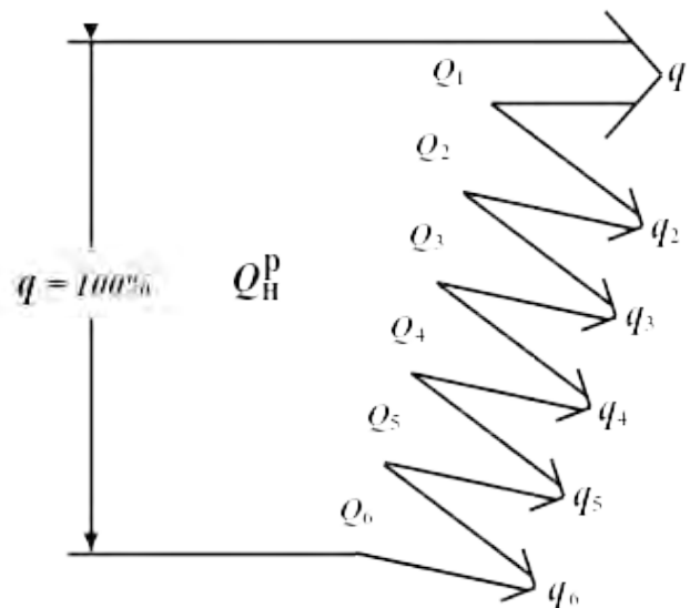
Рис. 4.2. Энергетическая диаграмма котла
